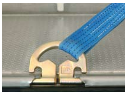
LS-ögla för surring på vänster sida. Surrning kan ske i olika vinklar. Enkel att montera vid öppna och stängda dörrar.
